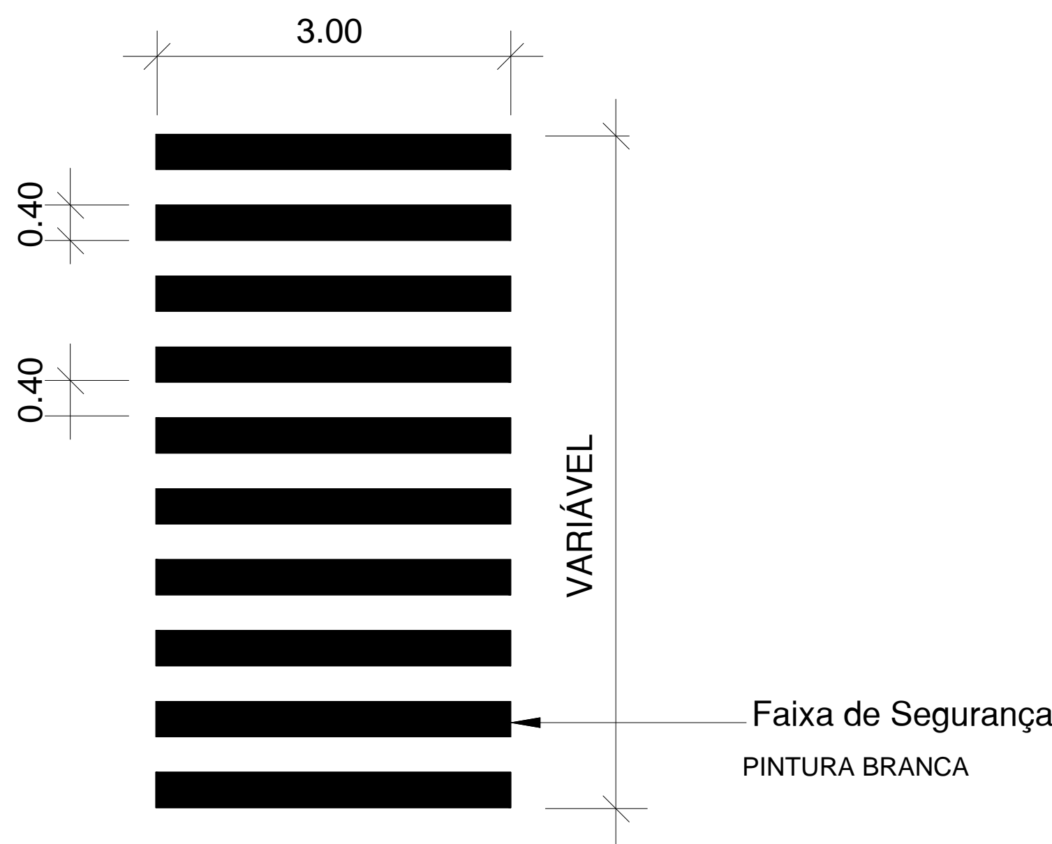
Detalhe - Faixa de Segurança e Retenção Sem Escala
