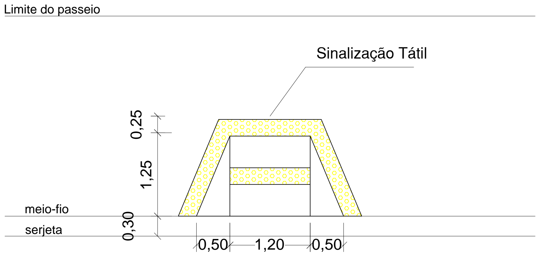
Detalhe - Rampa de Acessibilidade Sem Escala
